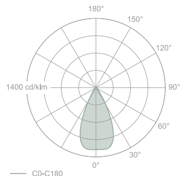
Krzywa światłości
