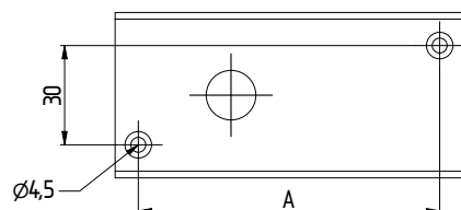
ROZSTAW OTWORÓW MONTAŻOWYCH OPRAWY [mounting holes spacing]
